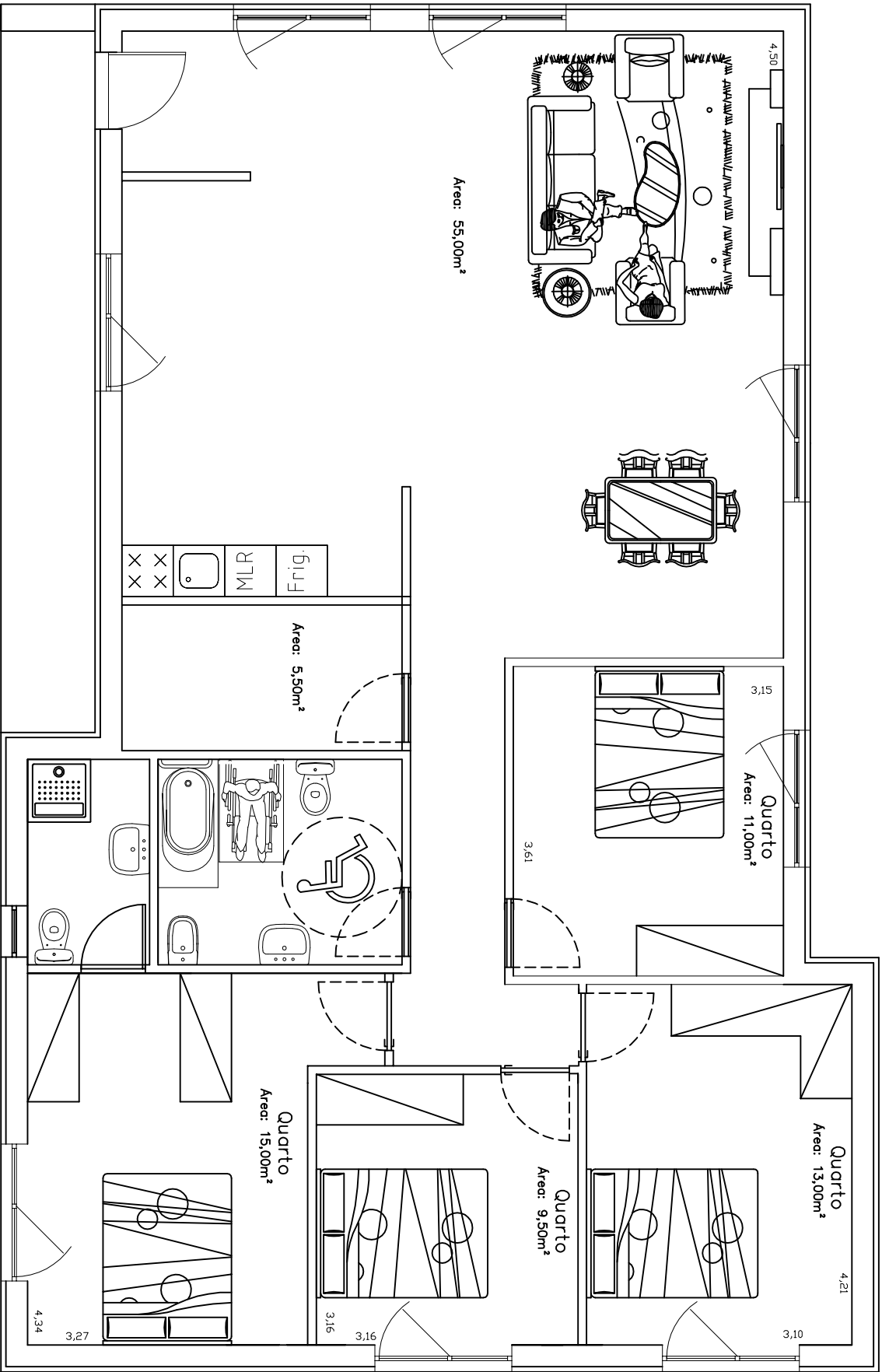
T3 Area de Implantação 155,00m²
